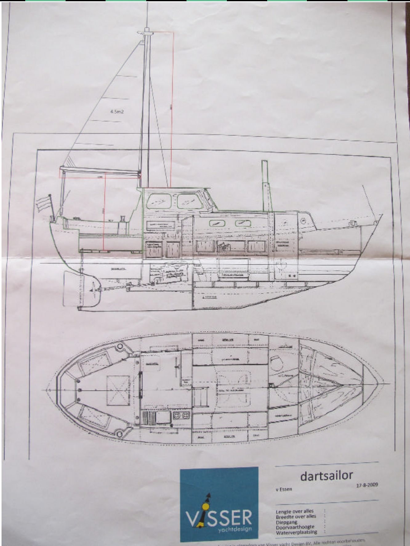
Ontwerptekening van de MATJE als motorkotter met korte mast
